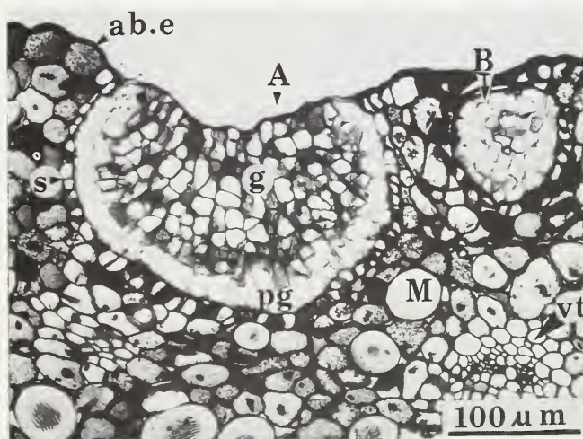
FIG. 2. 'n Dwarsdeursnee van volwasse, aktiewe klier. A: 'n mediane sneë; B: net aan die kant raakgesny ab. e: abaksiale epidermis; g: klierselle; M: mesofil; pg: perifere laag klierselle; s: skede; vr: vaatweefsel. (PAS & TB-kleuring).
